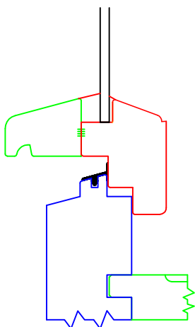
Variante 1 Einfachglas Ug-Wert ca 5,7 W/m 2 K
