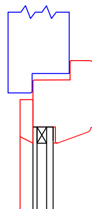
Variante 3 Iso 3-6-4 Ug-Wert 1,5 W/m 2 K mit Kryptonfüllung Ug-Wert 2,0 W/m 2 K mit Argonfüllung
