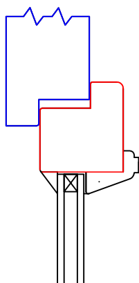
Variante 2 Iso 3-6-4 bis 3-14-4 Argonfüllung Ug-Wert 2,0 bis 1,1 W/m 2 K
