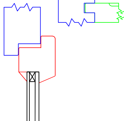
Variante 5 Iso 3-6-4 Ug-Wert 1,5 W/m 2 K mit Kryptonfüllung Ug-Wert 2,0 W/m 2 K mit Argonfüllung
