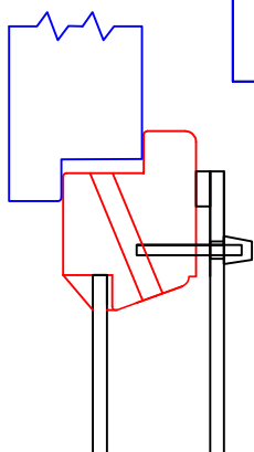
Variante 4 ESG-Vorsatzscheibe Ug-Wert ca 1,7 W/m 2 K
