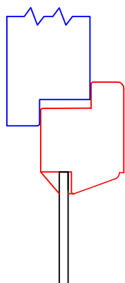
Variante 1 Einfachglas Ug-Wert ca 5,7 W/m 2 K
