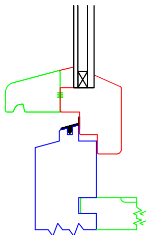
Variante 5 Iso 3-6-4 Ug-Wert 1,5 W/m 2 K mit Kryptonfüllung Ug-Wert 2,0 W/m 2 K mit Argonfüllung
