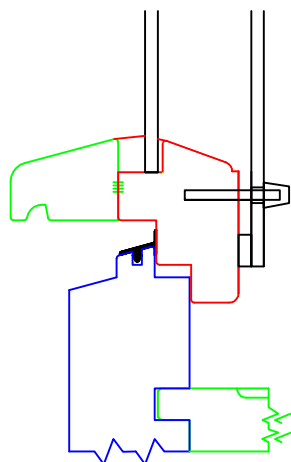
Variante 4 ESG-Vorsatzscheibe Ug-Wert ca 1,7 W/m 2 K
