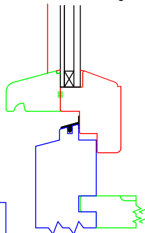
Variante 3 Iso 3-6-4 Ug-Wert 1,5 W/m 2 K mit Kryptonfüllung Ug-Wert 2,0 W/m 2 K mit Argonfüllung
