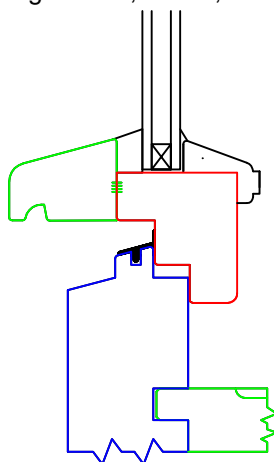
Variante 2 Iso 3-6-4 bis 3-14-4 Argonfüllung Ug-Wert 2,0 bis 1,1 W/m 2 K
